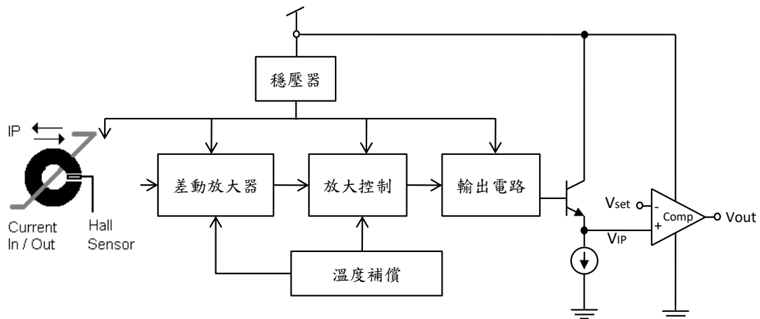
功能架構圖
